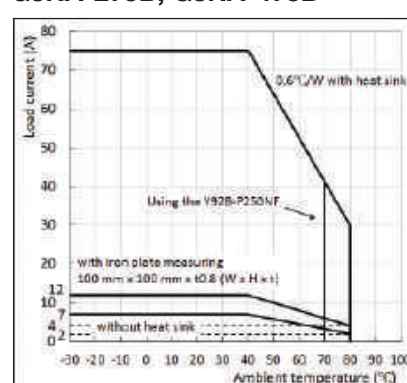
G3NA-275B, G3NA-475B
